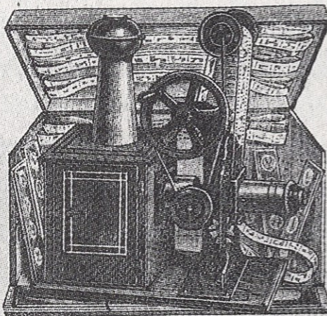
N° 19003. CINÉMATOGRAPHE lanterne magique, tôle lustrée. 0 m 33. 6 bandes, 6 verres . . . . 31. Le même, lanterne forte, 3 mèches . . . 43. CINÉMATOGRAPHE lanterne acajou, 12 verres, 6 bandes, 2 tableaux mécaniques . . . 17.50
