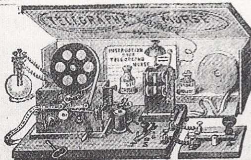
N° 1904. TÉLÉGRAPHE MORSE à mouvement d'horlogerie Petit modèle 37. | Grand modèle 57. TÉLÉGRAPHE BRÉGUET 4 postes. 21.50
