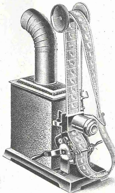
10/852/3 Kinematograph , mit Kondensor, Reflektor, Filmrolle und Schwungrad zur Transportregulierung, mit Petroleumlampe 3" Flachbrenner, 3 kurzen farbigen Filmen und 6 Glasbildstreifen 3 cm breit p. St. Mk. 15.—
