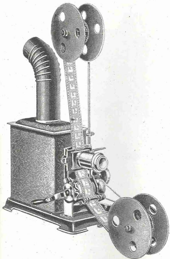
10/862/3 Kinematograph , mit Kondensor, Reflektor, 2 Filmrollen und Schwungrad zur Transportregulierung, mit Petroleumlampe 3" Flachbrenner, Aufpulvorrichtung, 3 kurzen, farbigen Filmen und 6 Glasbildstreifen 3 cm breit p. St. Mk. 18.—
