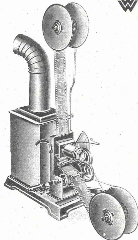
10/853/3 1/2 Kinematograph , mit Kondensor, Reflektor, 2 Filmrollen und Schwungrad zur Transportregulierung, mit Petroleumlampe 8" Flachbrenner, Bildeinstellvorrichtung, Aufpulvorrichtung, 3 kurzen, farbigen Filmen und 6 Glasbildstreifen 3 1/2 cm breit p. St. Mk. 30.—
